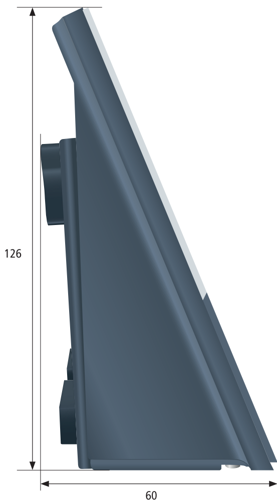
Indication de mesure en mm | Illustration 1:1
