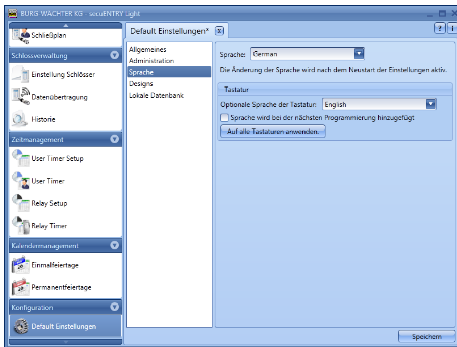
Abb. 53: Default Einstellungen Sprache
