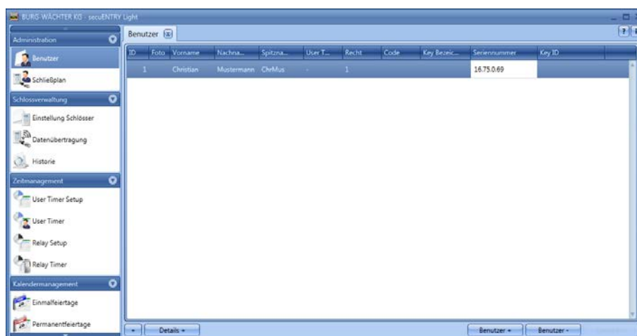
Abb. 68: Benutzerverwaltung
