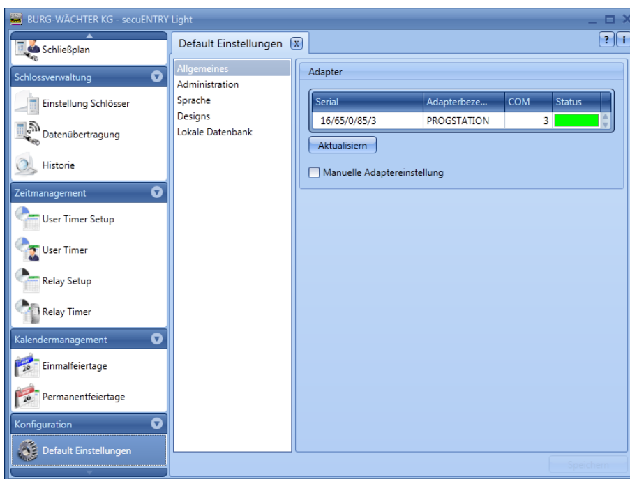
Abb. 50: Default Einstellungen
