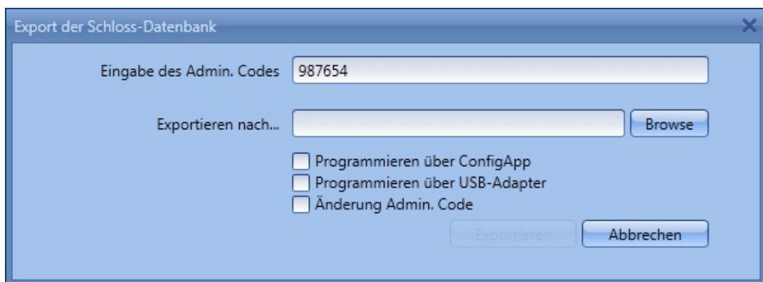
Abb. 89: Export Datenbank
