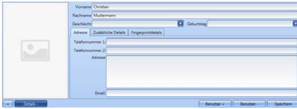
Abb. 56: Benutzerinformationen
