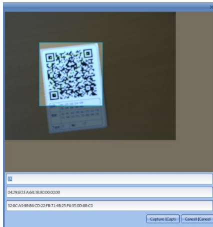
Abb. 64: QR-Code einscannen
