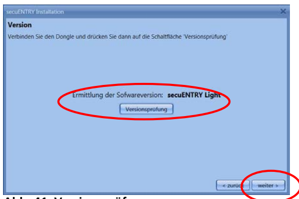
Abb. 41: Versionsprüfung
